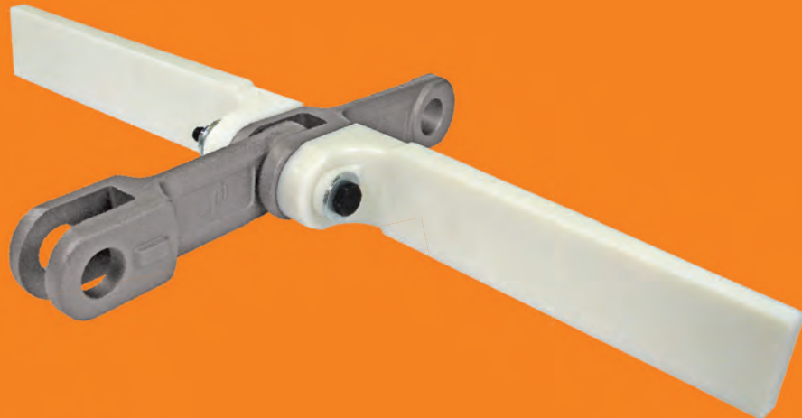
Bolt 'N' Go System ระบบสลัก 'N' Go
