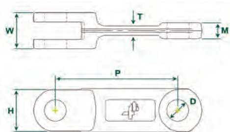
Standard Link ข้อต่อมาตรฐาน
