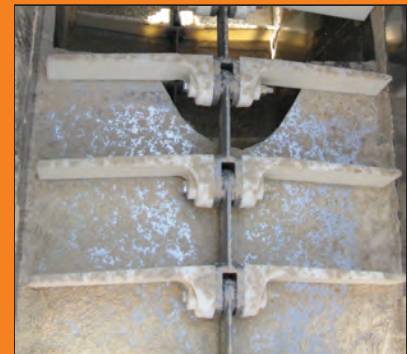
Feed Mill Application using Bolt 'N' Go Chain with Nylon Flights การใช้โซ่สลัก 'N' Go ที่ต่อเข้ากับปีกในลอน ในงานลำเลียงในโรงสี
