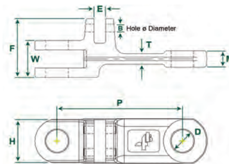
Double Link ข้อต่อแบบคู่
