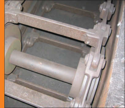
Typical Double Strand Chain Application ตัวอย่างการใช้งานโซ่มาตรฐานแบบคู่
