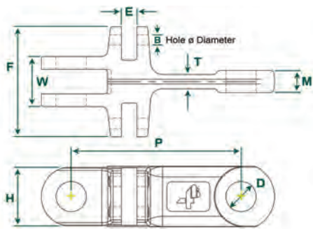
Triple Link ข้อต่อสามทาง
