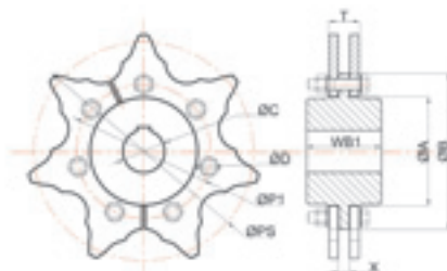
Reversibles Kettenrad (mit Bohrung)
