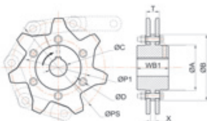
Standard Kettenrad (mit Bohrung)
